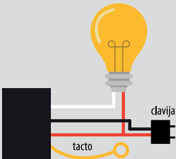
Diagrama de conexión SA-01.
