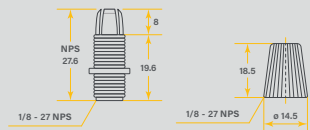
Sujetador para cable.
