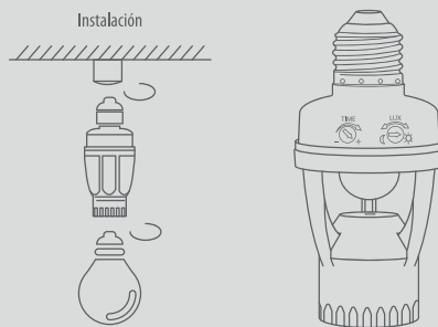
Portalámpara con sensor de movimiento 360°.
