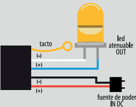
Diagrama de conexión SA-01L.
